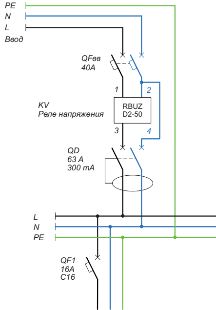
Схема 2. Вариант электрической схемы без транзита нуля через D2
