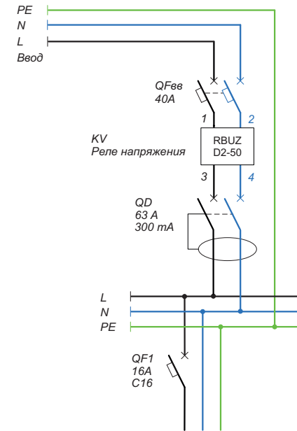
Схема 1. Вариант электрической схемы с транзитом нуля через D2
