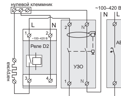
Схема 2. Подключение автоматического выключателя и УЗО без транзита нуля через реле
